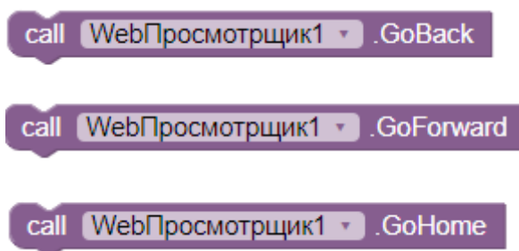
Рисунок 218. Вызов процедур перехода по ссылкам назад, вперед и домой
